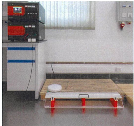
布置照片
