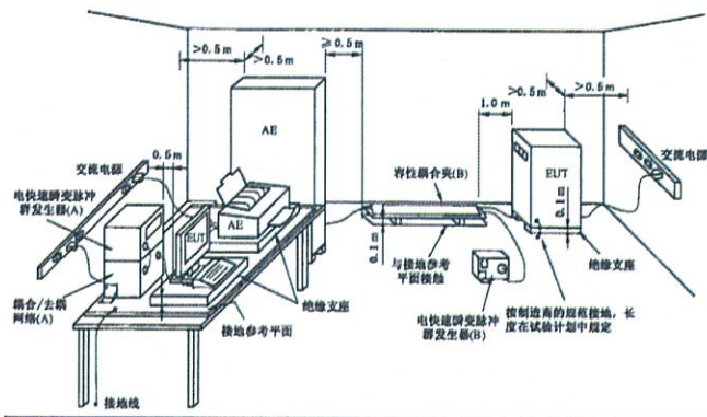
布置图
