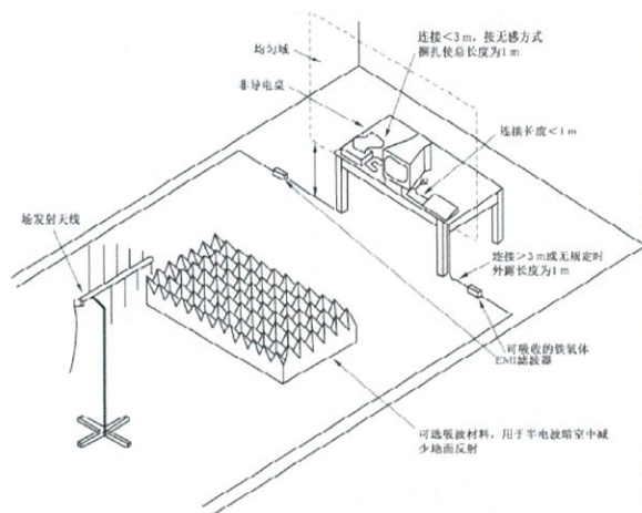
布置图
